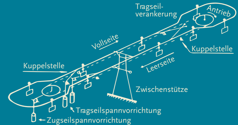
Schema einer Seilschwebbahn mit Umlaufbetrieb
